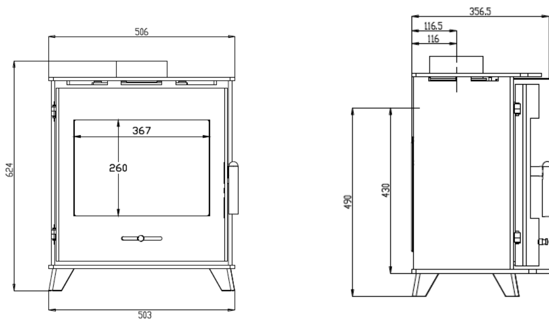
Technický výkres Newbourn 40:
