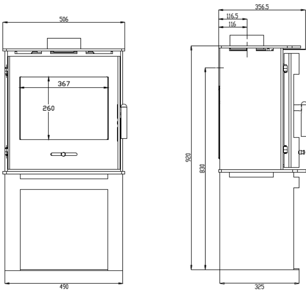
Technický výkres Newbourn 40S:
